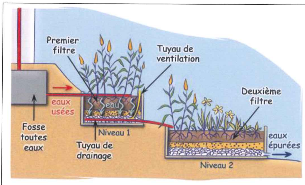
Schéma de principe de la phytoépuration
