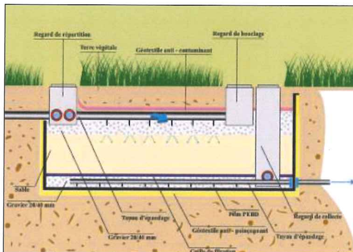
Lit filtrant vertical drainé
