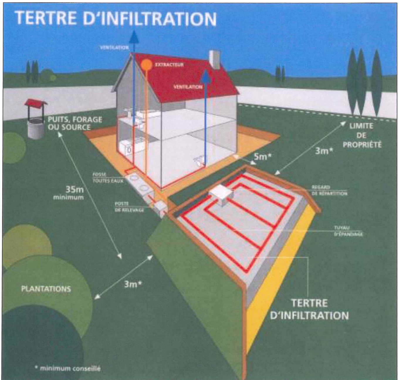
Schéma de principe du terre d'infiltration
